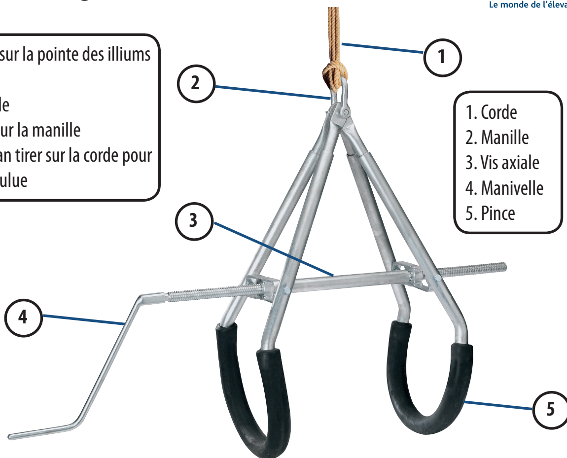
Visuel A: Élévateur gros bovins, gris - schéma technique
